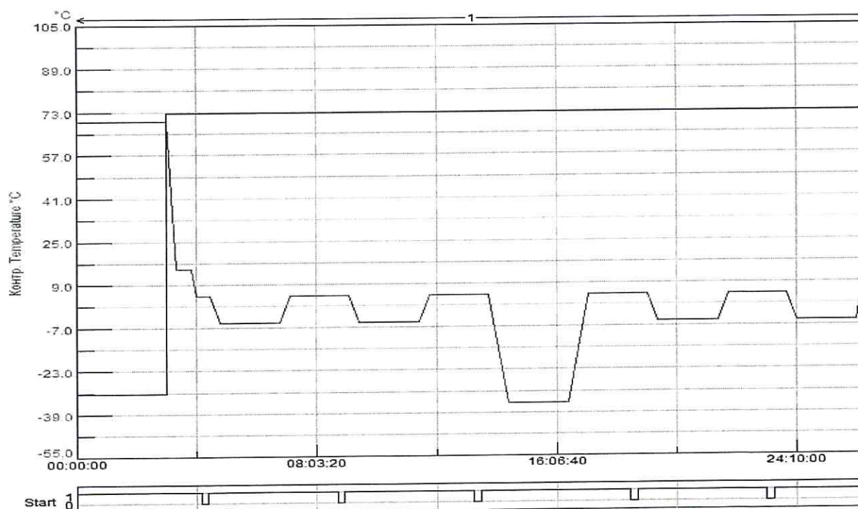
Рисунок А.1 – Графическая модель одного цикла климатических испытаний
