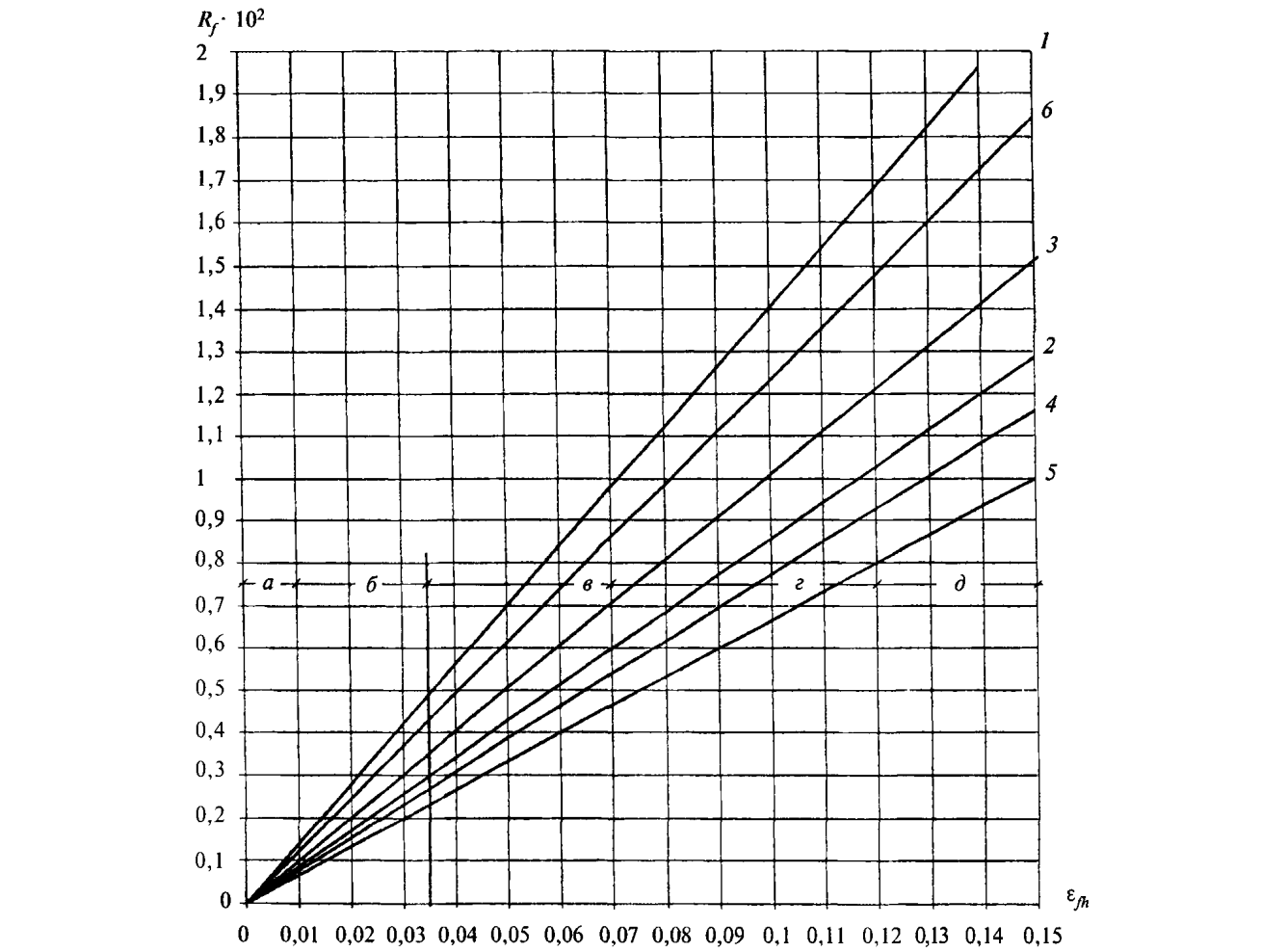
1, 2 — супеси; 3 — суглинки; 4 — суглинки с 0,07 < I_p \leq 0,13 ; 5 — суглинки с 0,13 < I_p \leq 0,17 ; 6 — глины (в грунтах 2,4 II 5 содержание пылеватых частиц размером 0,05 — 0,005 мм составляет более 50 % по массе); а — практически непучинистый; б — слабопучинистый; в — среднепучинистый; г — слабопучинистый; д — чрезмернопучинистый
