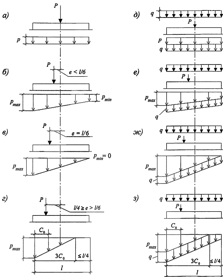
а-г – при отсутствии нагрузок на полы; д-з – при сплошной равномерно распределенной нагрузке интенсивностью q ; а и д – при центральной нагрузке; б и е – при эксцентриситете нагрузки e < l/6 ; в и ж – при e = l/6 ; г и з – при e > l/6 (с частичным отрывом фундамента от грунта)
