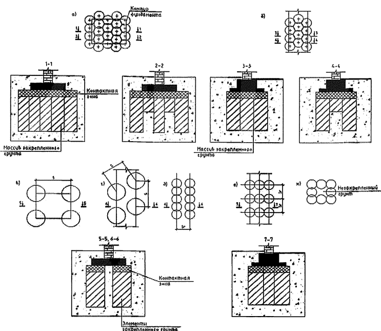
а, б – сплошное из рядом расположенных элементов; в, г – отдельно стоящих элементов; д, е, ж – отдельно расположенных рядов сплошных элементов
